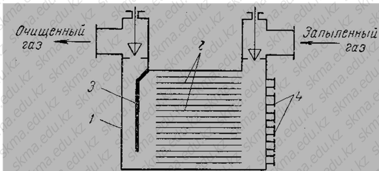
Рис. 8.6 Пылеосадительная камера: 1 – камера; 2 – горизонтальные перегородки (полки); 3 – отражательная перегородка; 4 – двери.
