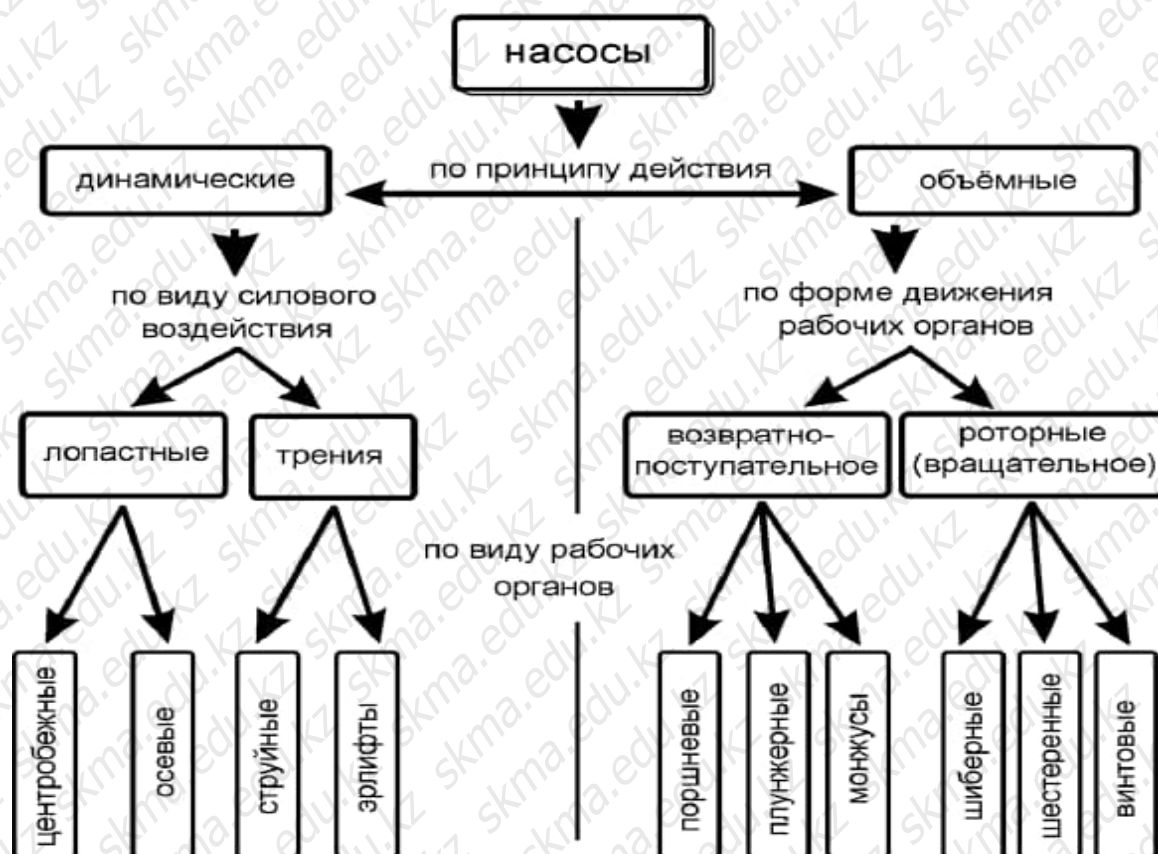
Рисунок 1 Классификация насосов
