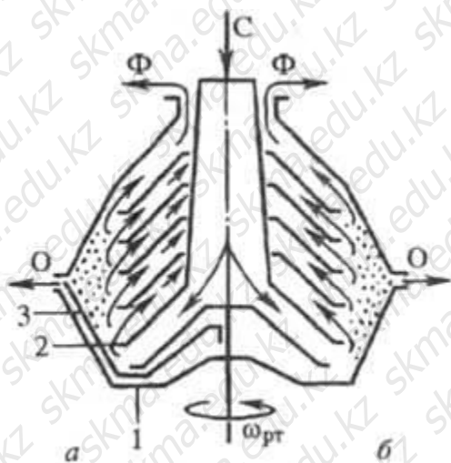
Рис. 3. Сепараторы для разделения суспензий: на рис. совмещены сепаратор-очиститель (а) и сепаратор-сгуститель (б); 1 - ротор; 2 - пакет тарелок; 3 - подвижное днище.
