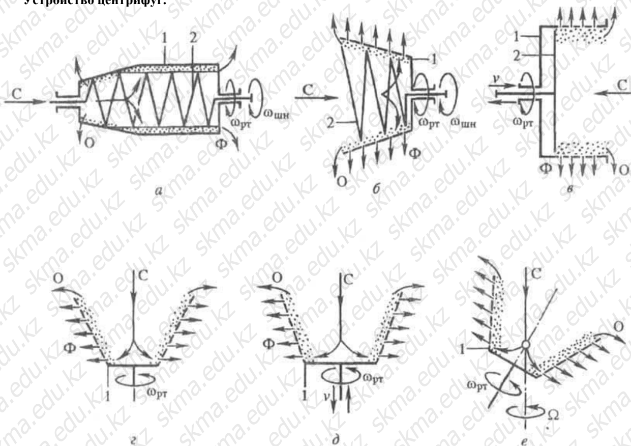
Рис. 2. Центрифуга непрерывного действия: а - осадительная шнековая; б - фильтрующая шнековая; в - с пульсирующей выгрузкой осадка; г - инерционная; д - вибрационная; е - прецессионная; 1 - ротор; 2 - механизм выгрузки.
