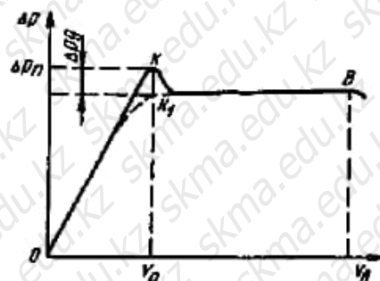
Рисунок 2. Кривая псевдоожижения
