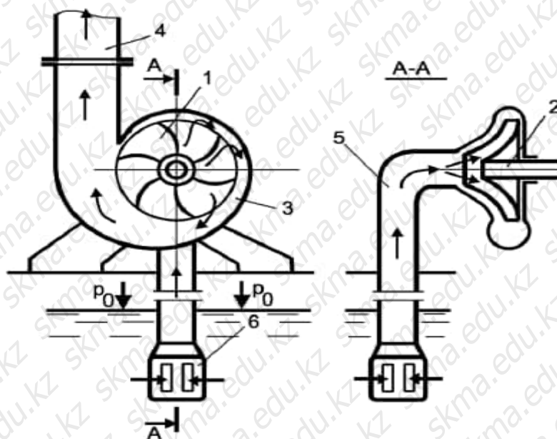
Рис. 4.3 Центробежный насос
